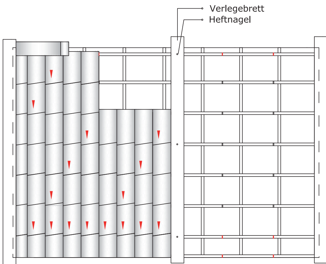
Schneenasenanordnung jeder 3. Dachstein
