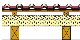
LINITHERM PAL 2U auf Sparren, Gipsfaserplatten unter Sparren
