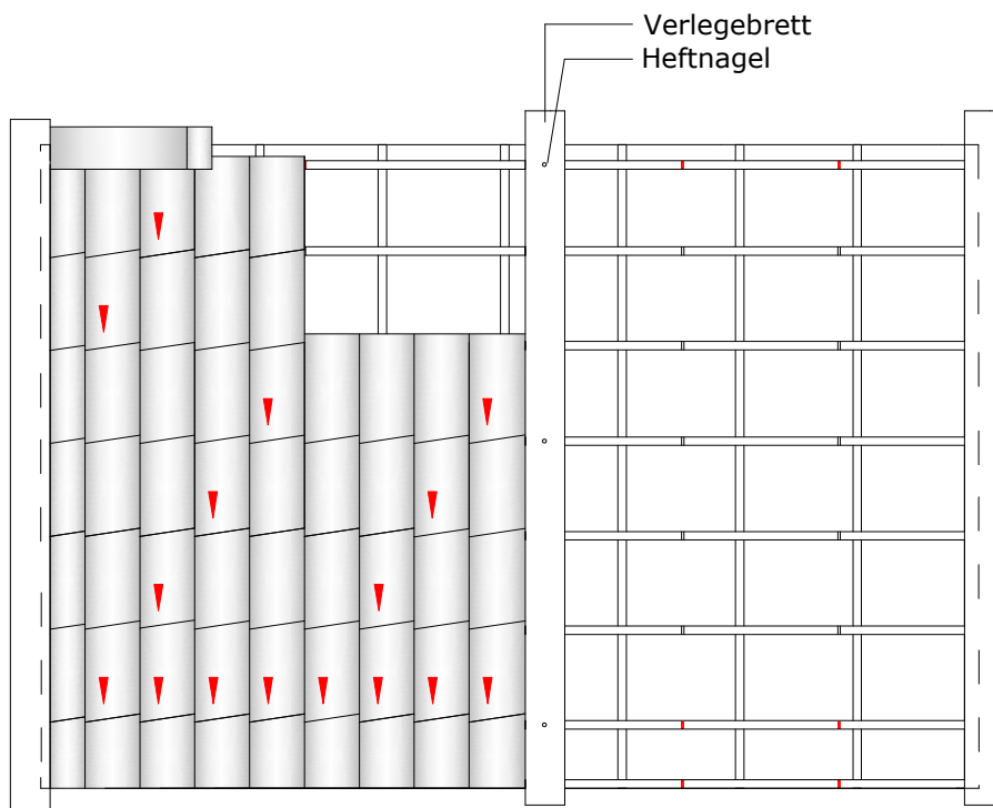
Schneenasenanordnung jeder 3. Dachstein
